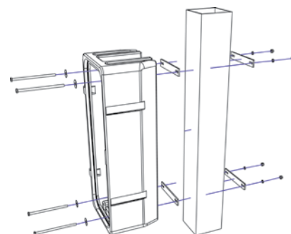
Fixing points / Points de fixation / Montagepunkte / Puntos de montaje
